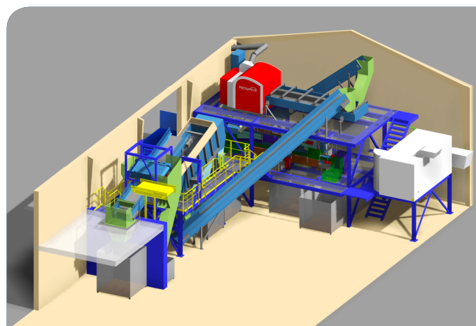
3D oversigt over plastsorteringslinje fra REDWAVE
